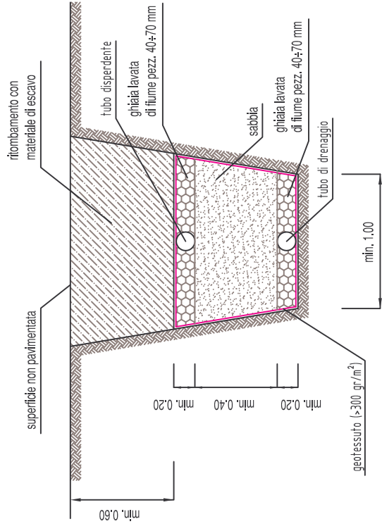
SEZIONE TRINCEA CON FILTRO A SABBIA
